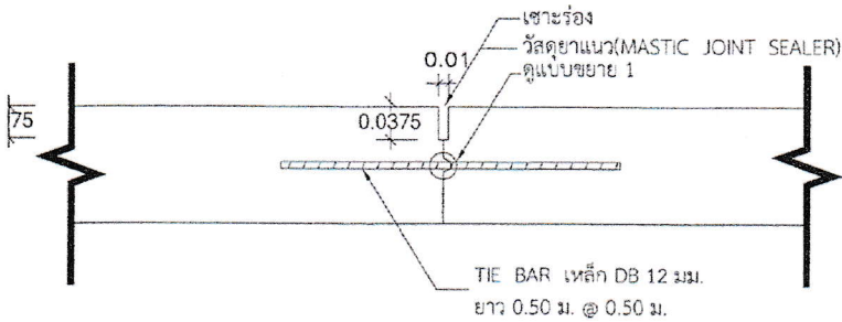
แบบขยายรอยต่อ LONGITUDINAL JOINT
